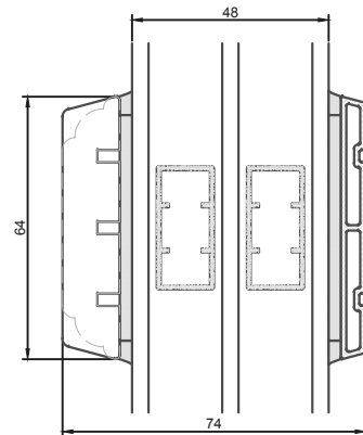
64 mm vandret energisprosse
