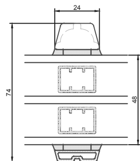
24 mm lodret energisprosse
