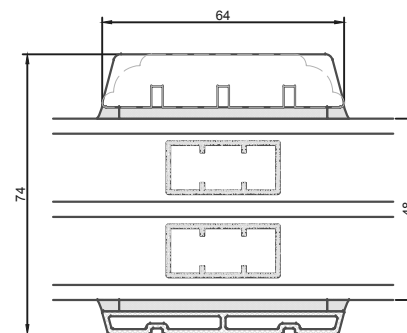
64 mm lodret energisprosse
