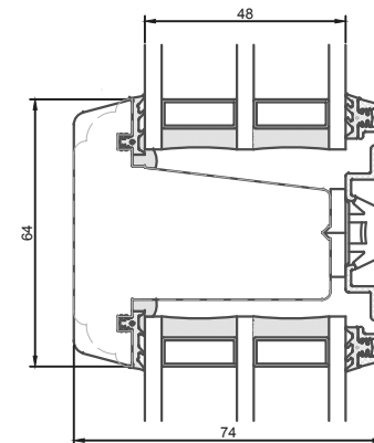
64 mm vandret sprosse
