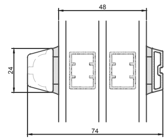
24 mm vandret energisprosse
