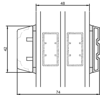
42 mm vandret energisprosse
