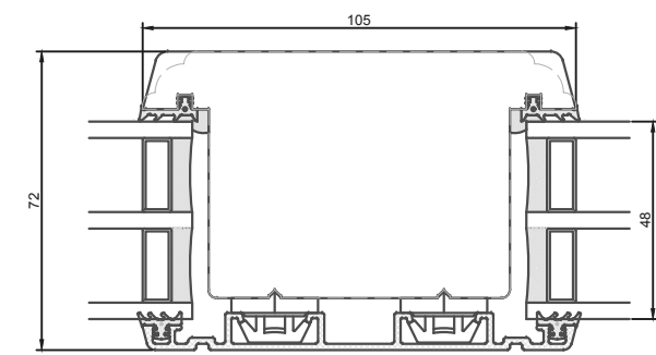
105 mm lodret tapstykke
