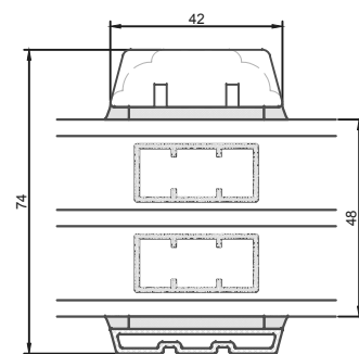
42 mm lodret energisprosse
