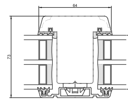
64 mm lodret sprosse
