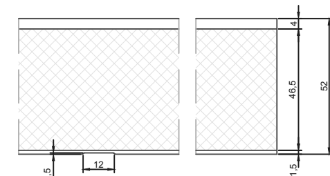
Snit B-B
