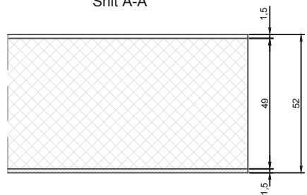
Snit A-A
