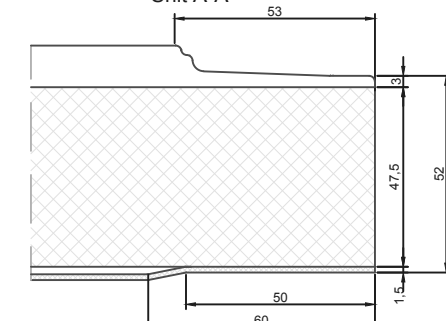
Snit A-A
