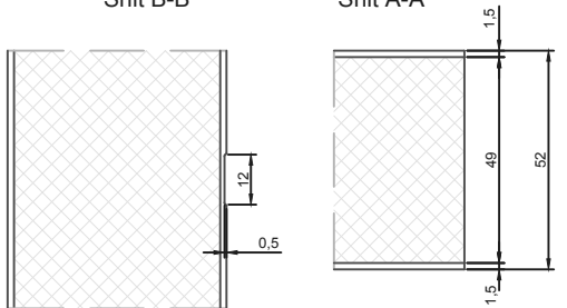
Snit B-B
