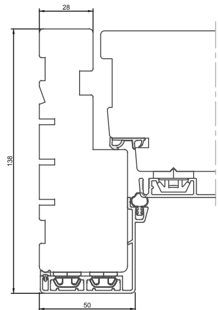
138 mm karm - indadgående dør
