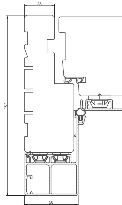
167 mm karm - indadgående dør
