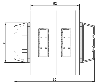
42 mm vandret energisprosse
