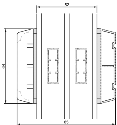
64 mm vandret energisprosse
