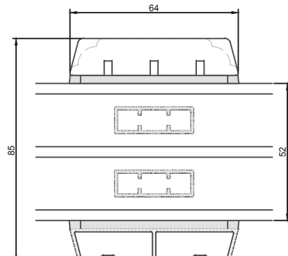
64 mm lodret energisprosse
