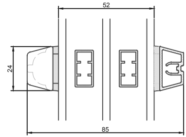
24 mm vandret energisprosse
