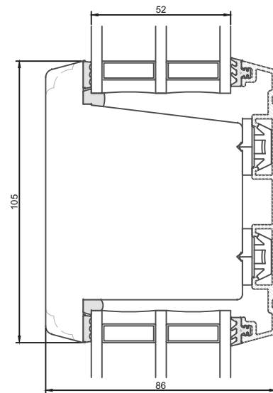
105 mm vandret tapstykke
