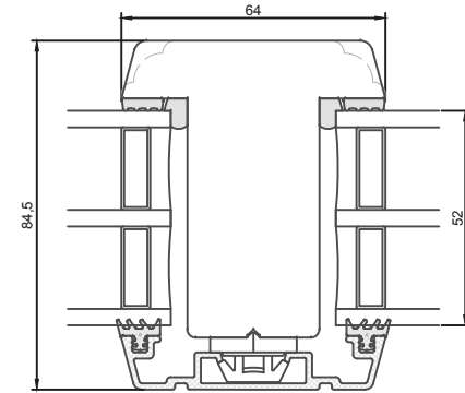
64 mm lodret prosse
