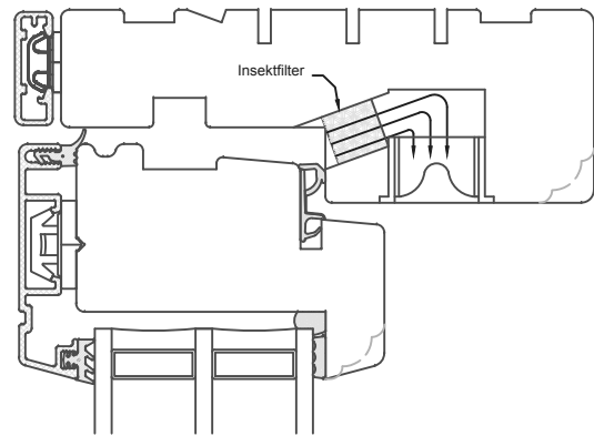
Klikventil på udadgående vindue med aftræk i fals
