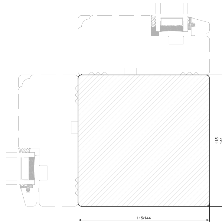
90° samling med stolpe
