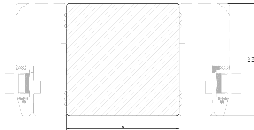
180° samling med stolpe
